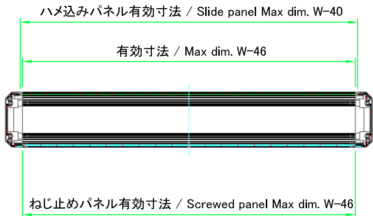
A-A (1:5)
